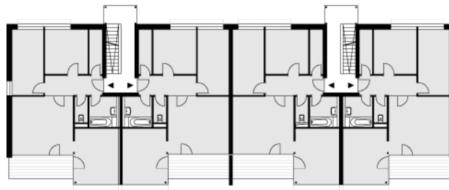
1. Obergeschoss - Objekt B,C,D,E
