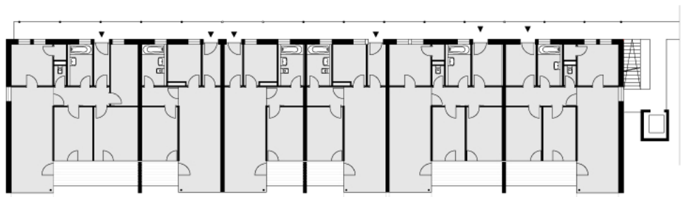
1. Obergeschoss - Objekt A
